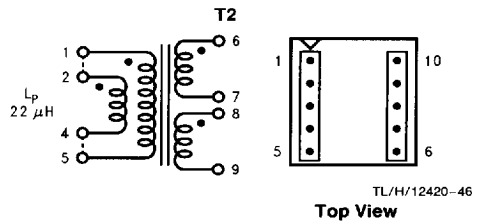
FIGURE 30. Schott 67140860
