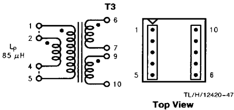
FIGURE 31. Schott 67140920
