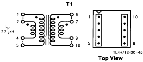
FIGURE 29. Schott 67141450
